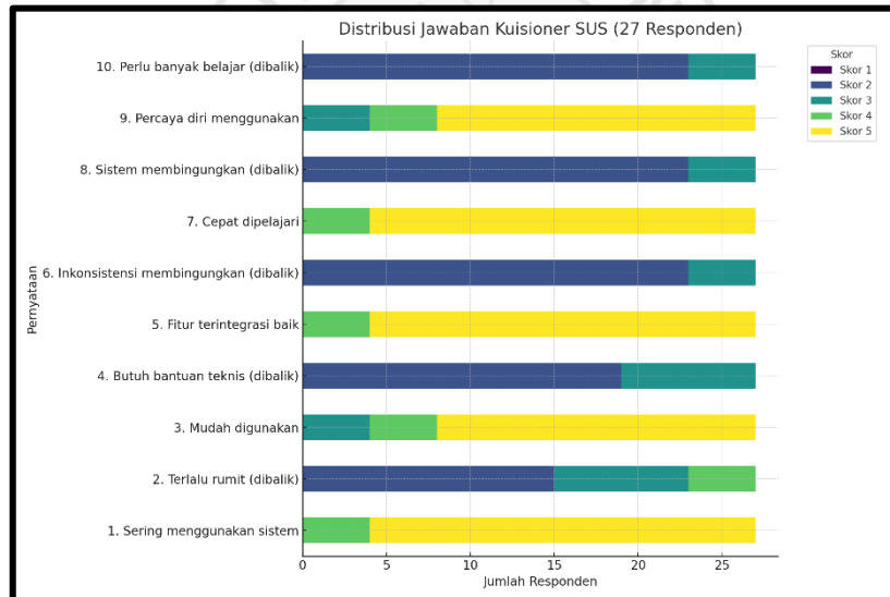
Gambar 4. Diagram Hasil Pengujian SUS
