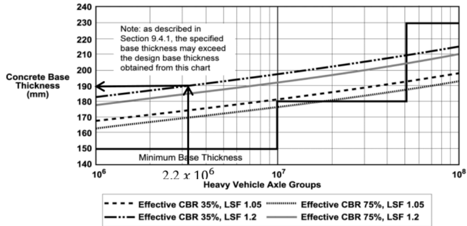
Gambar 4. 3 Grafik desain contoh perkerasan beton polos tanpa sambungan dowel (Sumber: Hasil analisa (2025))
