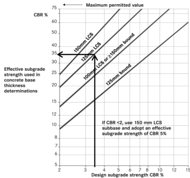
Gambar 4. 2 Peningkatan kekuatan tanah dasar efektif dengan lapisan subbase terikat (Sumber: Hasil analisa (2025))
