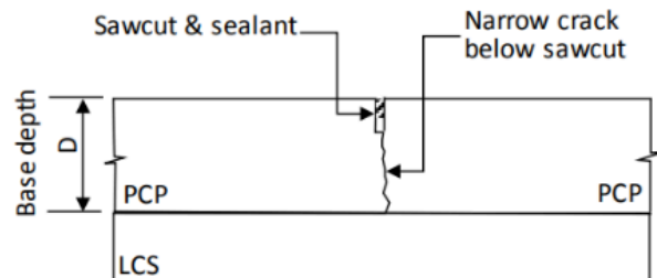
Gambar 2. 13 Contoh sambungan kontraksi transversal yang digergaji pada PCP (Sumber: Guide to Pavement Technology Part 2 (2017))
