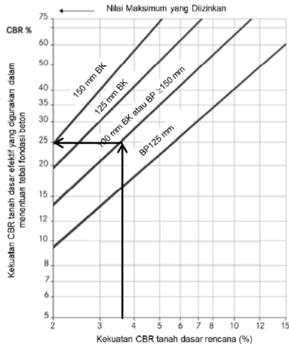
Gambar 4. 1 CBR tanah dasar efektif dan tebal pondasi bawah
