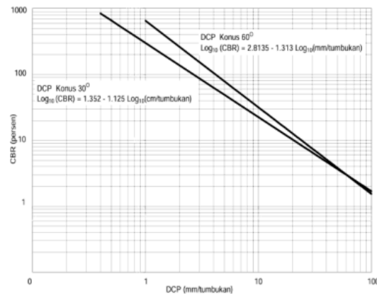
Gambar 2. 19 Hubungan nilai DCP dengan CBR)
