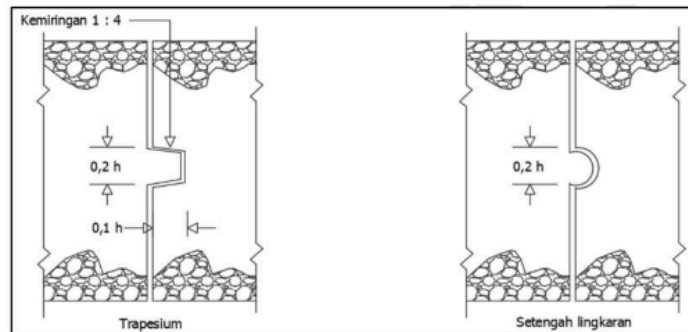
Gambar 2. 5 ukuran standar penguncian sambungan memanjang (Sumber: Manual Desain perkerasan jalan (2024))
