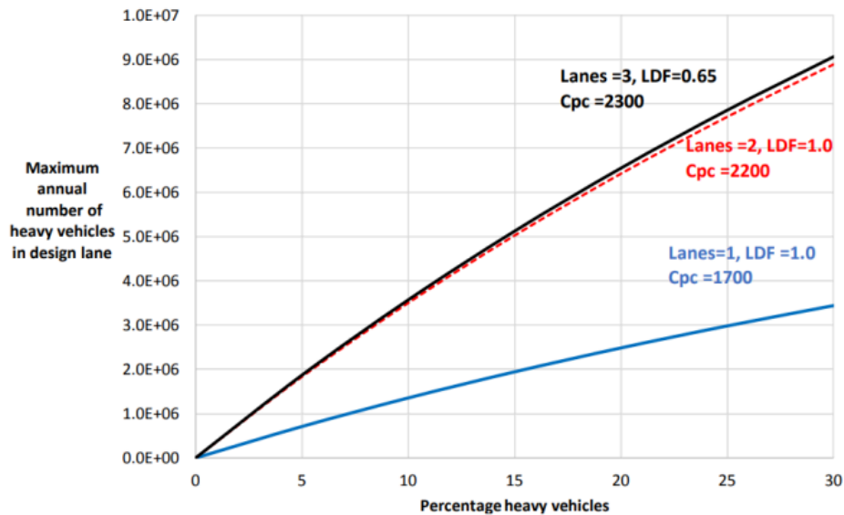
Gambar 2. 8 Jumlah maksimum kendaraan berat tahunan di jalur desain untuk E_{HV} = 2 (Sumber: Guide to Pavement Tecnology Part 2 (2017) )
