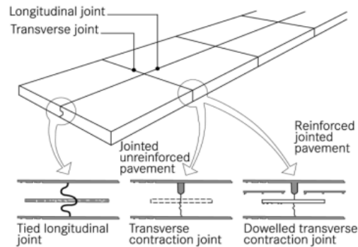
Gambar 2. 12 Sambungan khas pada perkerasan jalan beton (Sumber: Guide to Pavement Technology Part 2 (2017))
