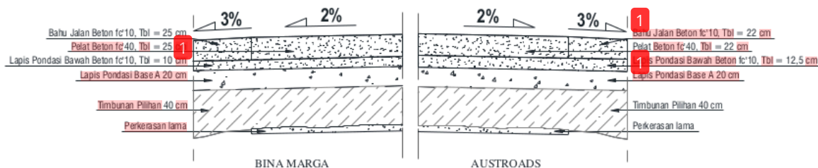
Gambar 4. 4 Detail Potongan Melintang (Sumber: Hasil analisa (2025))
