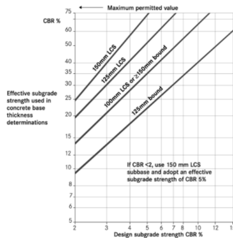
Gambar 2. 9 Peningkatan kekuatan tanah dasar efektif dengan lapisan subbase terikat atau beton kurus (LCS)
