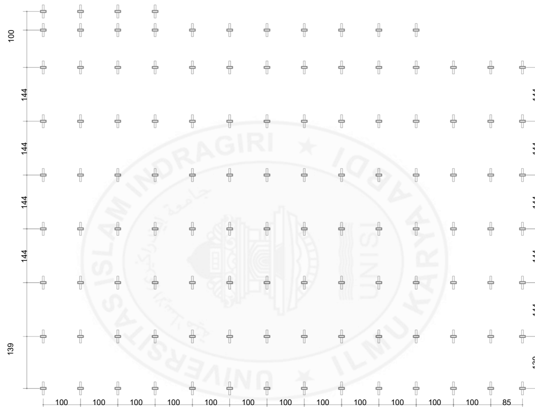
DENAH PONDASI TONGKAY KAYU ULIN
