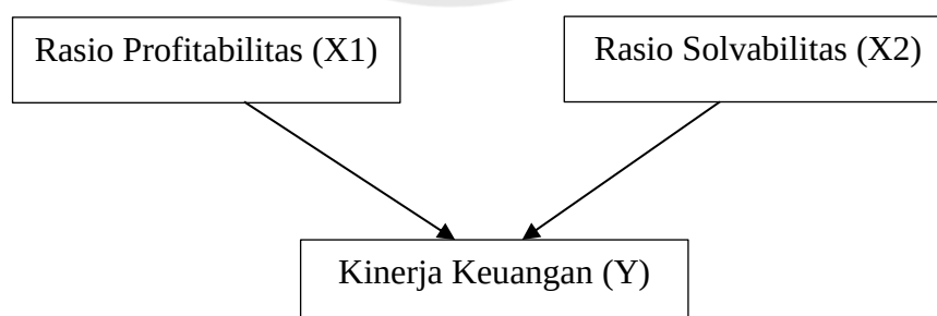
Gambar 2.1 : Kerangka Pemikiran
